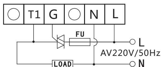
ZKD-2A调整器接线图
