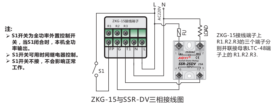
ZKG-15与SSR-DV三相接线图
