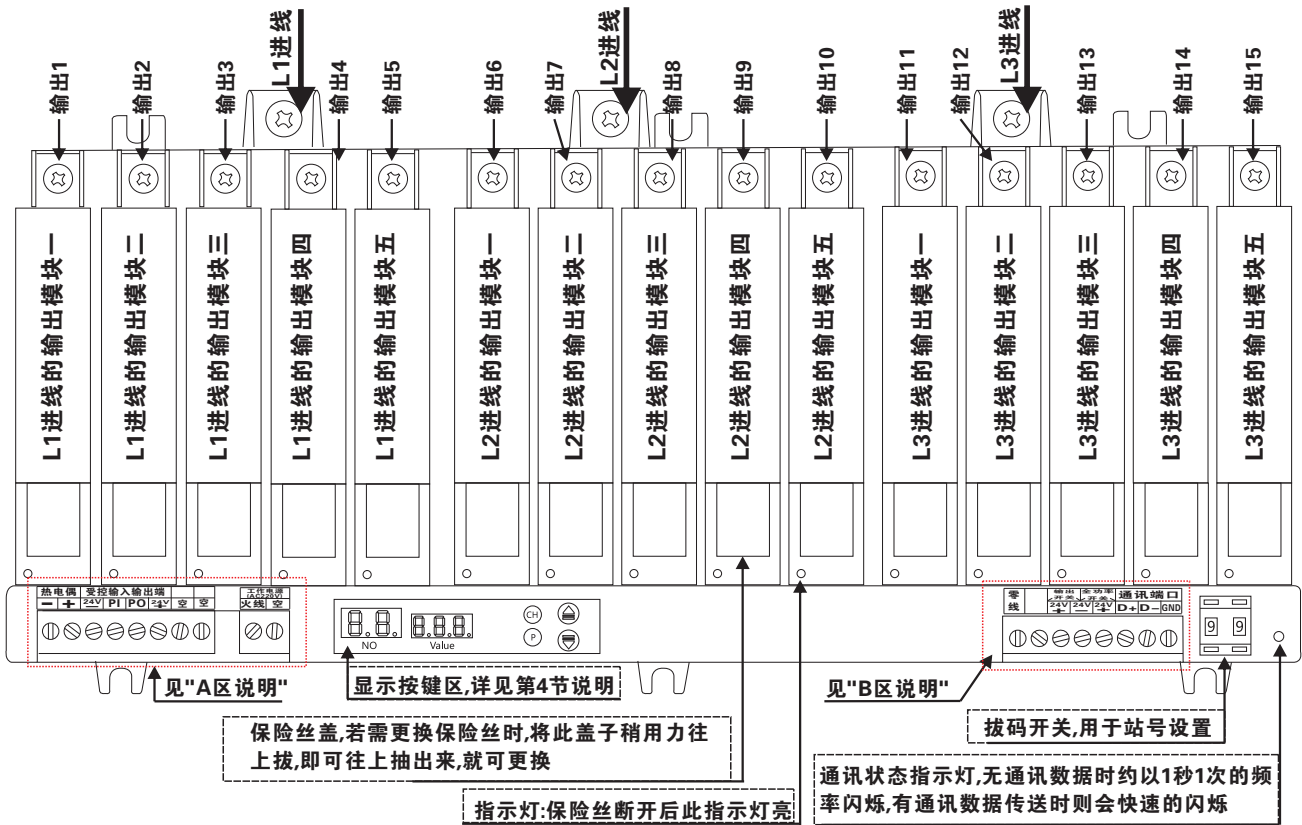
图4:模块功能分布图及说明
