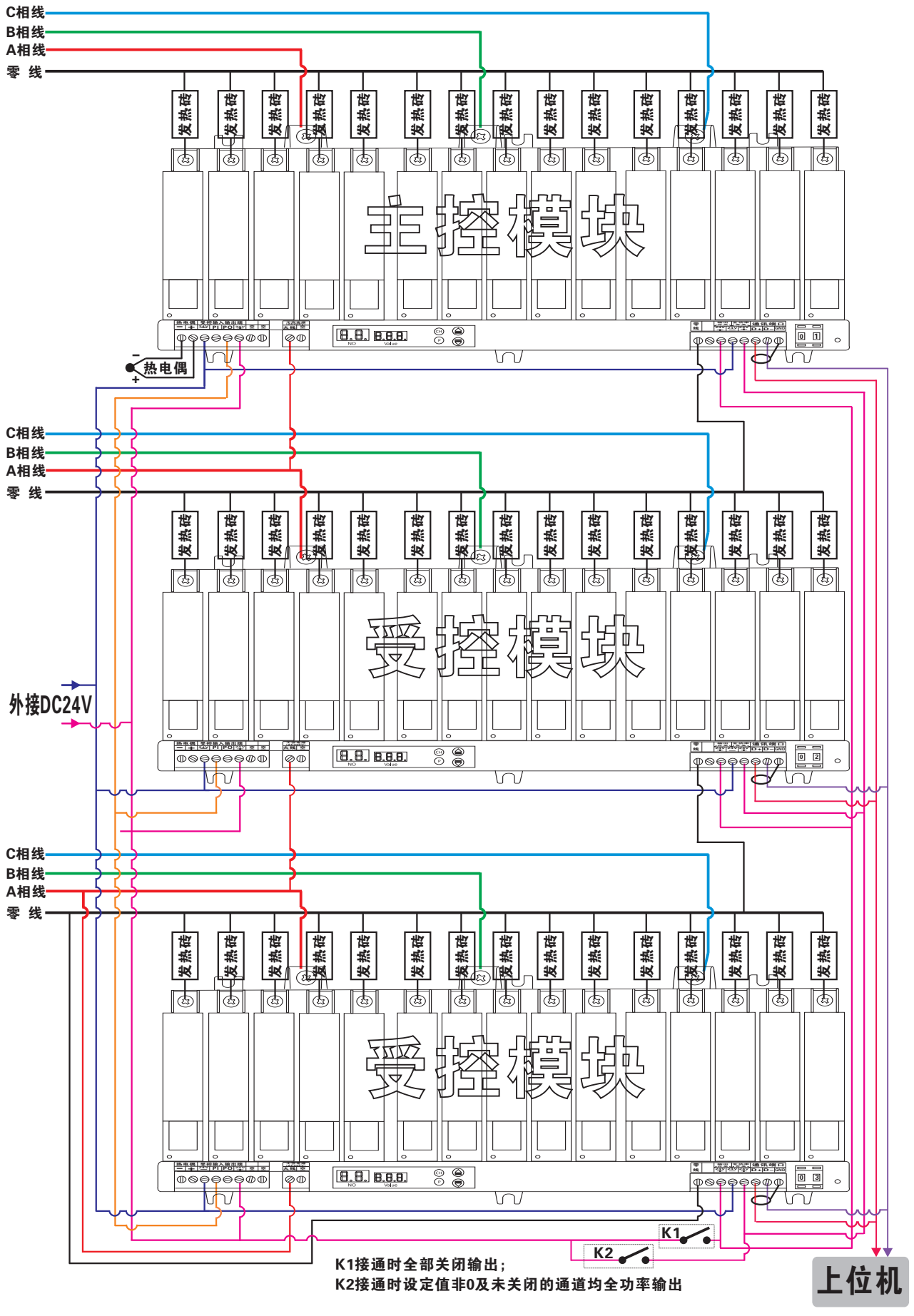
图5:三块模块联动受控接线实例图（限于篇幅，多块模块接法类同）
